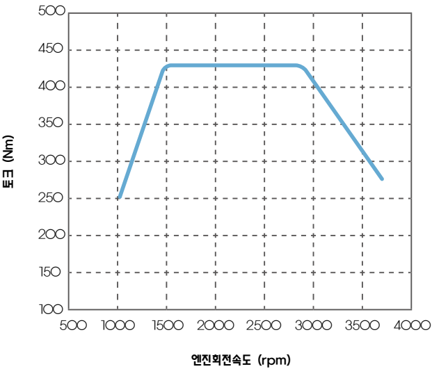
F1C VGT 180 토크 성능곡선
