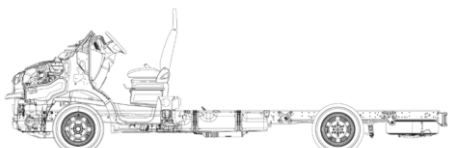
Versione scudato ridotto CCS
